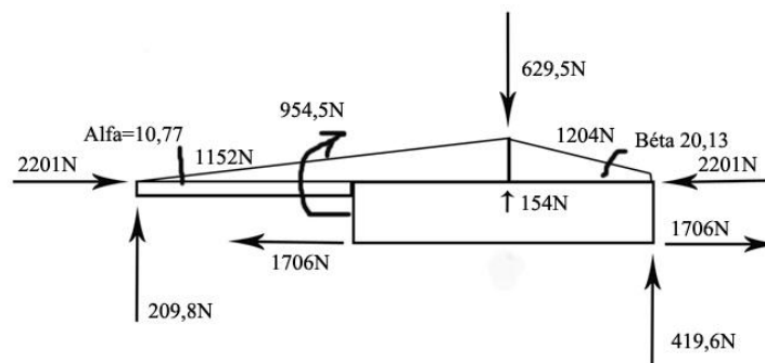
51. ábra Egy négyhúros \frac{3}{4} -es nagybőgő sematikus erőtanai ábrázolása. Láthatók a húrok húzóerői (1152N), a tető nyomó- (2201N) illetve a hát húzóerői (1706N), a szemöldökök támaszerői (209,8N és 419,6N), a lábon át a tetőre jutó nyomóerő (629N), a tetőre a tető domborulata miatt kialakuló felfelé ható erő (154N). Végül a nyakhajlatban a húrok húzóerejéből támadó forgatónyomaték (954,5N). A mértékegység N=Newton, 10N=1 kg.
