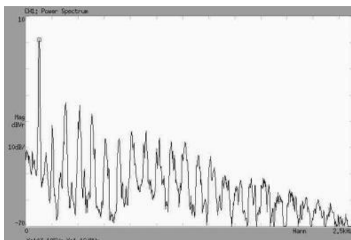
44. ábra A Man-Mo100-gl4 ráfelelési görbéje.
